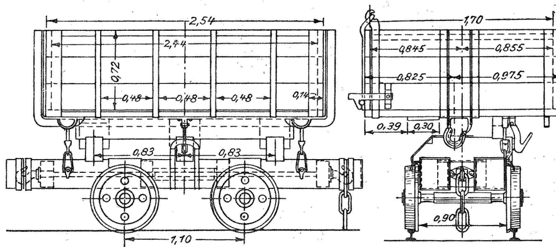
Bild 121. Holzkastenkipper, 900 mm Spur, 3m 3 Inhalt
